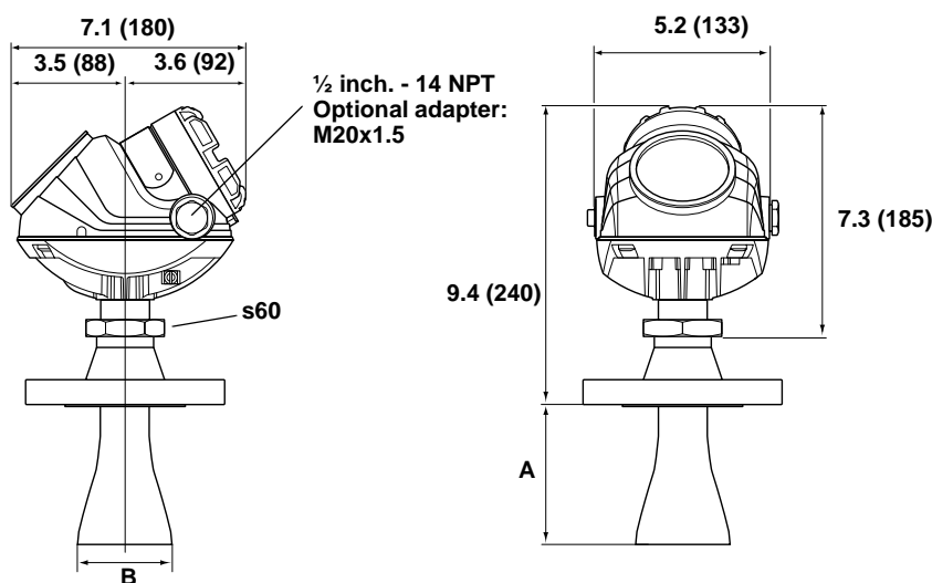
5402 Dimensions
